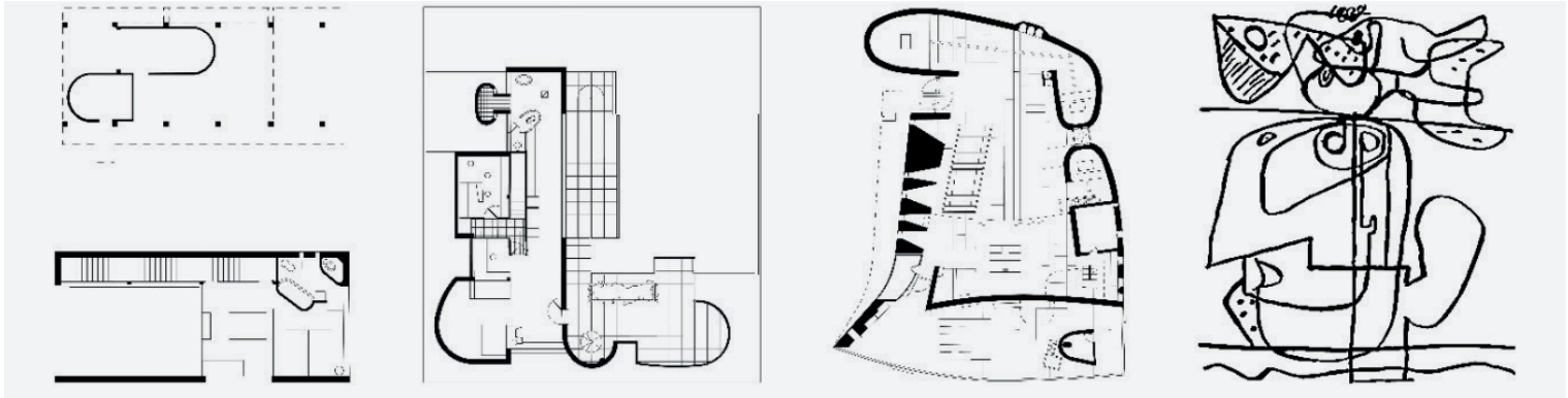
Figura 1. De izquierda a derecha: Casa Citrohan, plantas; Villa Savoye, planta terraza jardín; Capilla de Ronchamp, planta baja; Taureau, pictograma. Fuente: Elaboración propia, 2025.
