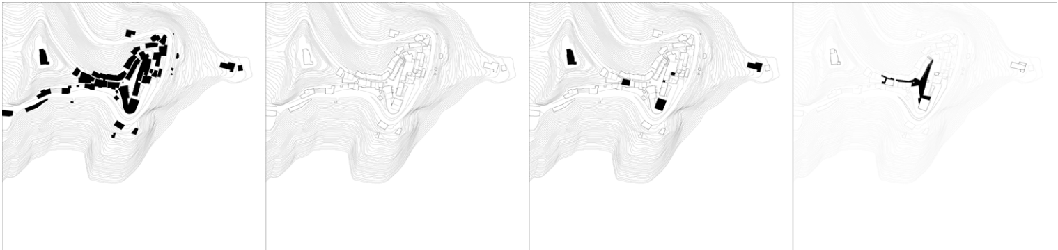
Figura 2. Arquata del Tronto: la morfología del pueblo, los emergentes arquitectónicos y el espacio de la plaza. Fuente: Investigación coordinada por Luigi Coccia y Sara Cipolletti.
